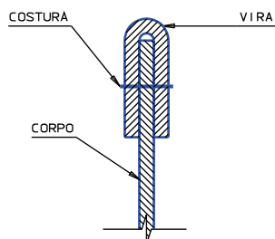
DETALHE - ARREIMATE TÍPICO
