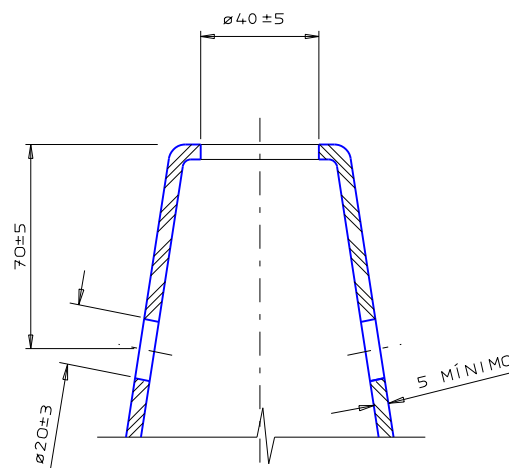
CORTE A-A
