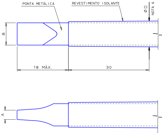
DETALHES DA PONTA
