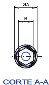
CORTE A-A
