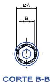
CORTE B-B
