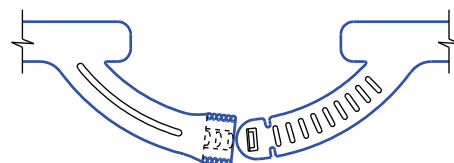
SISTEMA DE AJUSTE DA CARNEIRA ALTERNATIVA 1 (NOTA 4)
