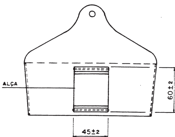
VISTA POSTERIOR
