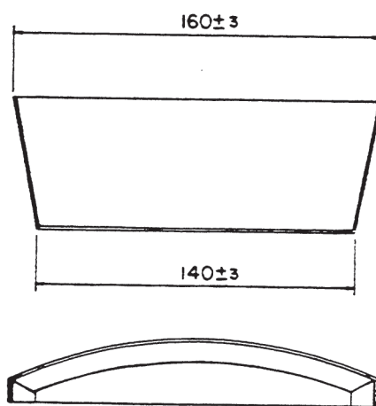
ARMAÇÃO (NOTA 3)
