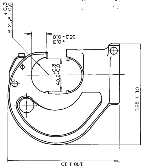
CABEÇOTE - PEÇA 1 DETALHE SEM COBERTURA ISOLANTE
